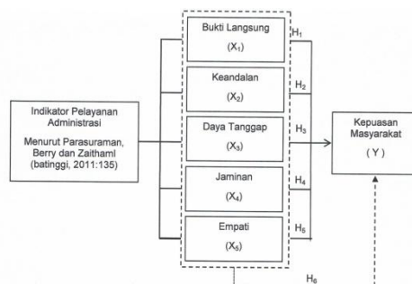
Gambar 1 : Kerangka Pemikiran
