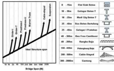
Gambar. 3. Bentang ekonomis jembatan
