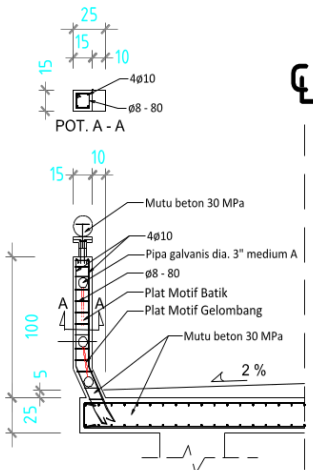
Gambar. 5. Detail penulangan tiang sandaran dan pelat lantai jembatan
