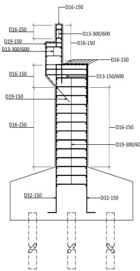
Gambar. 7. Detail penulangan abutmen yang digunakan adalah 11 meter, dengan diameter 30 cm dan jarak antar tiang adalah 90 cm, gambar detail dimensi pondasi dan penulangan tersaji pada tampilan Gambar 8.
