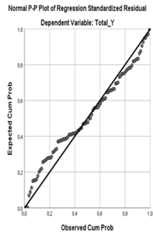
Gambar 2 Hasil Uji Normalitas
