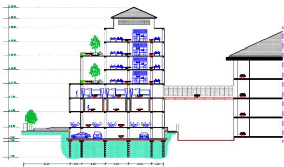
Gambar 10. Gambar Potongan membujur
