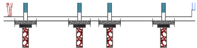
Gambar 14. Gambar Pondasi Sumuran
