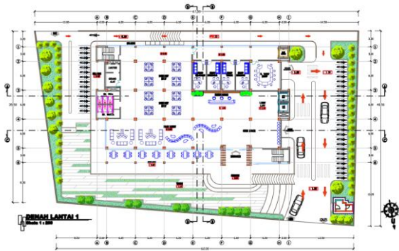
Gambar 7. Gambar denah lantai dasar Bangunan
